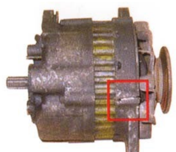
PRASKLÝ DRŽÁK
